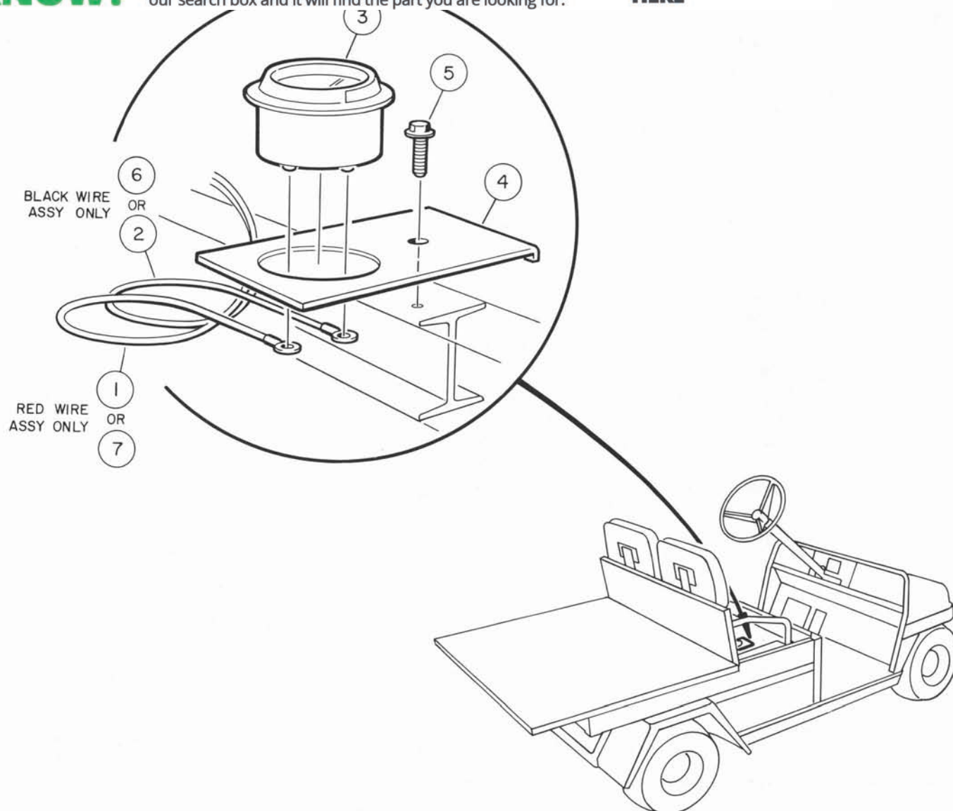
FIGURE 7-18. HOUR METER KIT — 36 VOLT. SEE LIST 7-18.
